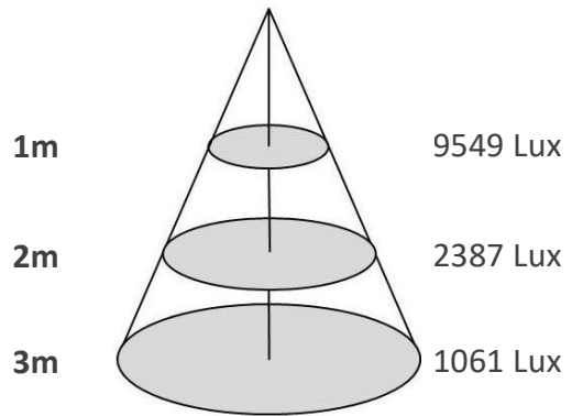
UFO-HB3-C-150W.lux
